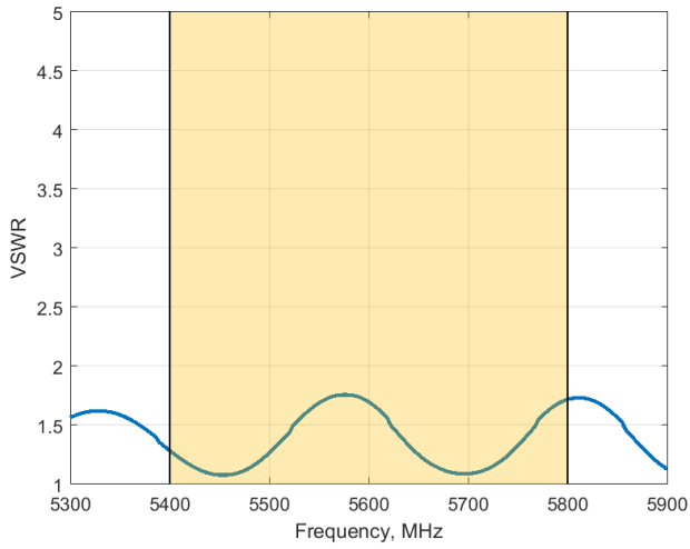
VSWR 5000-6000 MHz
